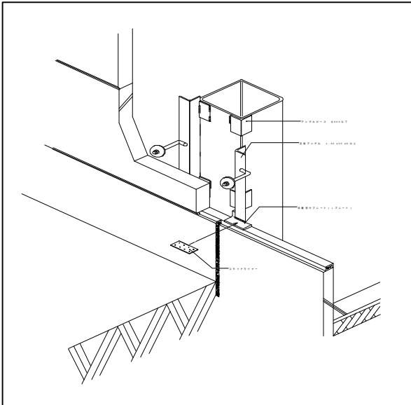
横ボルトP-2
