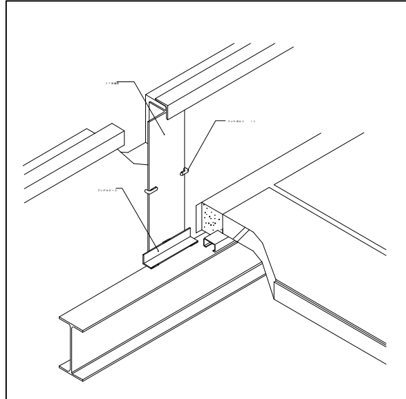
横ボルトP-3
