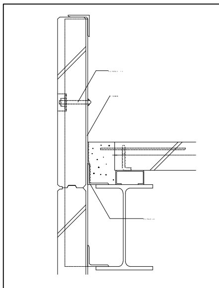
横ボルト - 4
