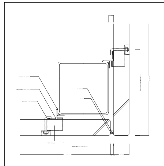
横ボルト - 6
