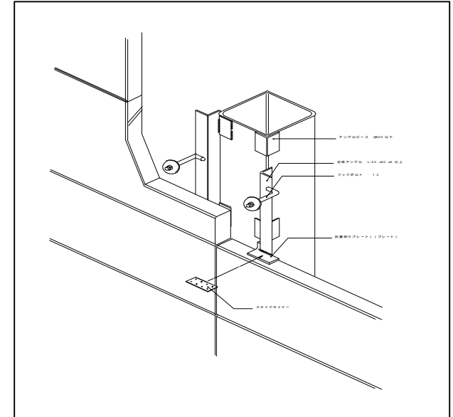
横ボルトP-1
